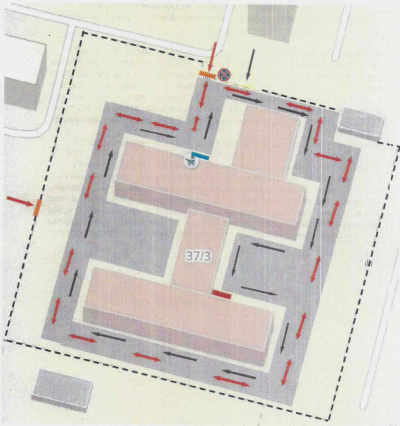
3. План—схема движения транспортных средств по территории МБДОУ детский сад №78 «Ивушка» к месту разгрузки/погрузки и рекомендуемые безопасные пути передвижения воспитанников
